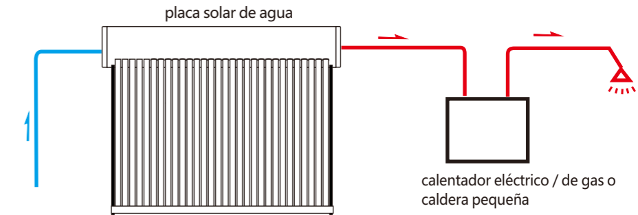
Esquema con calentadores de agua eléctricos o a gas, o con calderas pequeñas.
